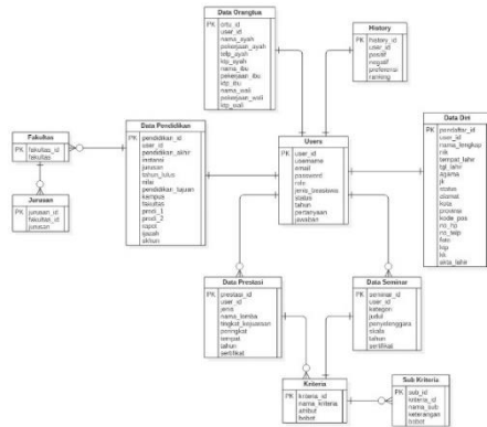
Gambar 9. Rancangan ERD
